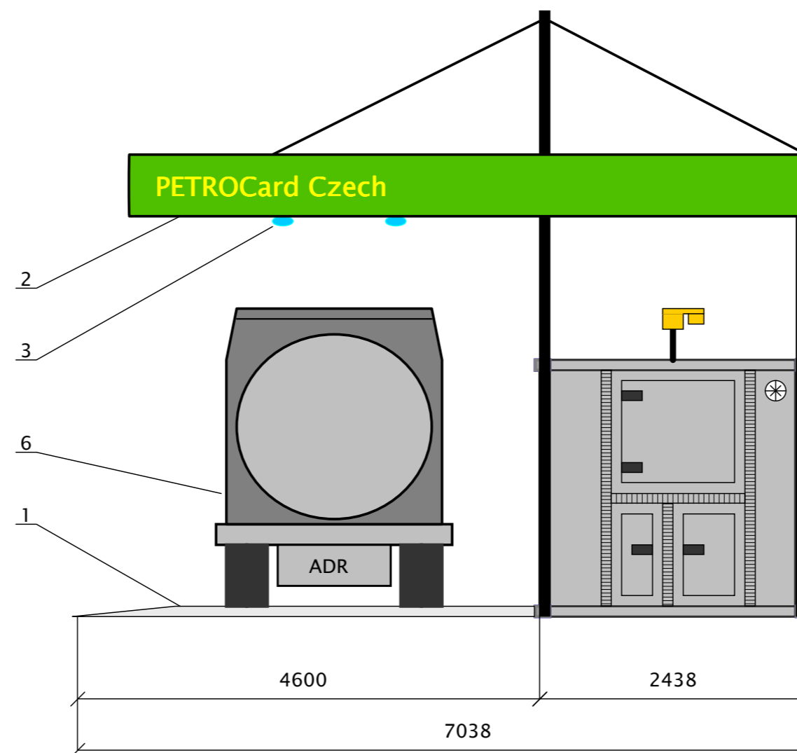
Čelní pohled
